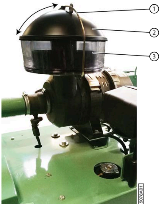
Fig. 101: Nettoyer l'avant filtre
