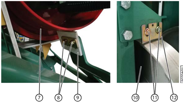
Fig. 92: Régler les racleurs
