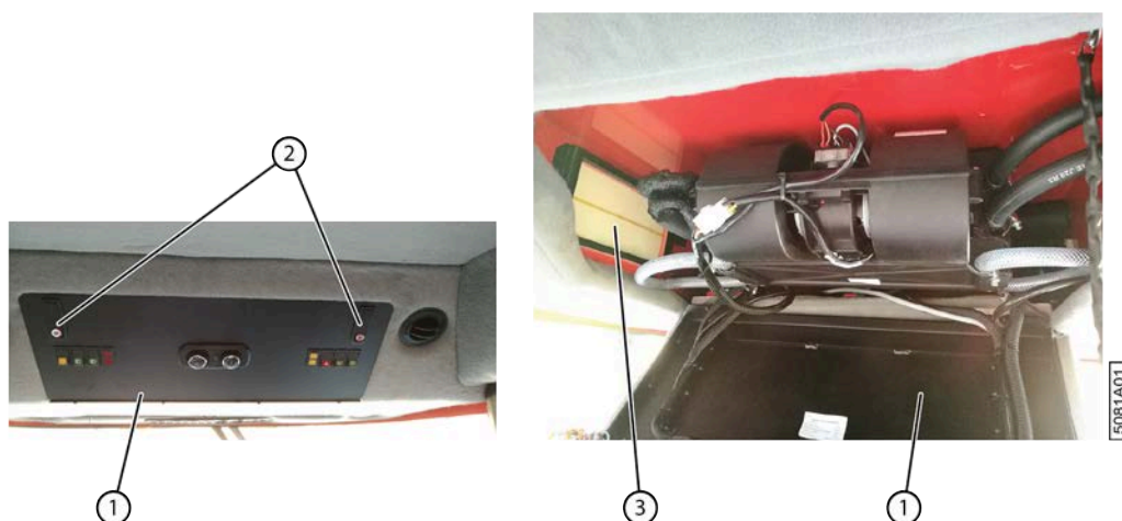
Fig. 106: Filtre à air dans le plafond de la cabine
