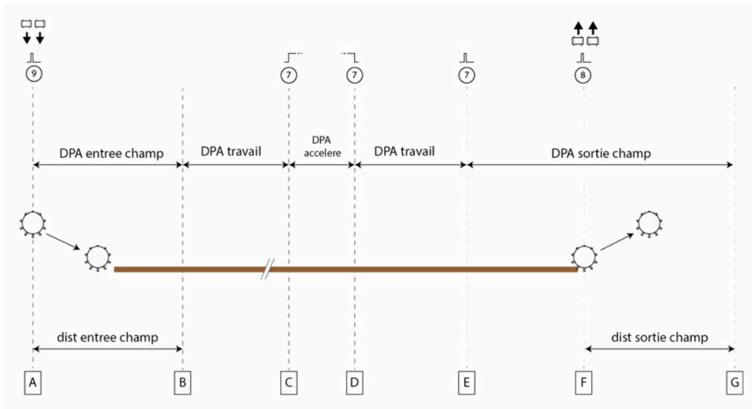
Fig. 78: DPA et distance pendant le rodage et l'épandage
