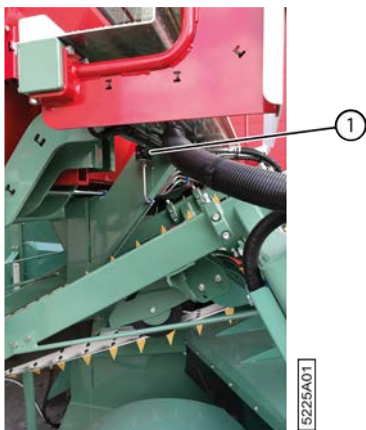
Fig. 115: Filtre d'aération du réservoir à carburant
