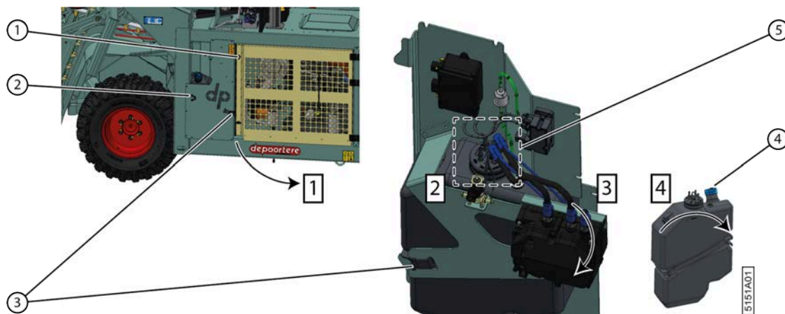
Fig. 135: Démontez et vidanger le réservoir d'AdBlue
