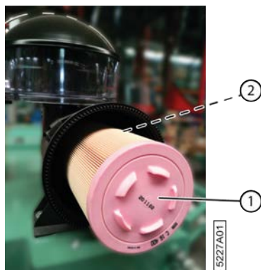
Fig. 137: Élément principal et élément de sécurité du filtre à air
