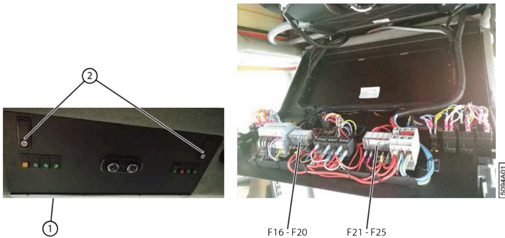
Fig. 127: Remplacer un fusible dans la cabine
