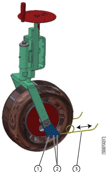
Fig. 88: Réglages possibles de la roue de jauge
