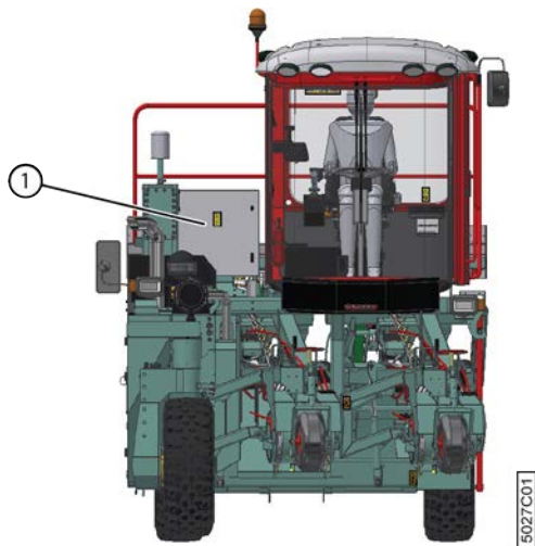
Fig. 29: Armoire électrique
