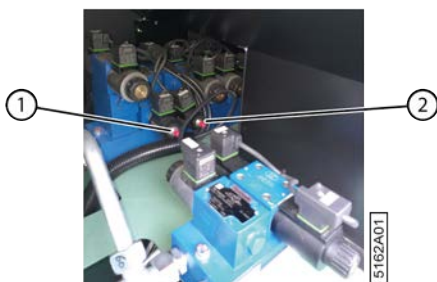
Fig. 80: Commande manuelle
