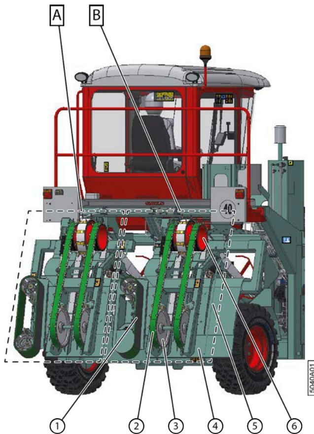
Fig. 34: Zone de dépôt
