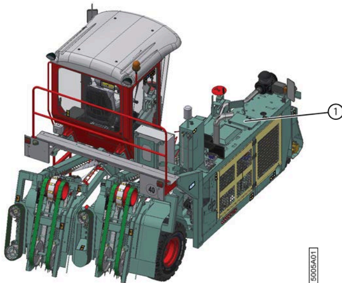
Fig. 37: Emplacement de la boîte à outils
