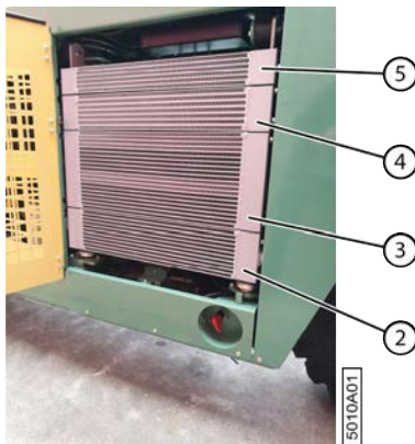
Fig. 102: Nettoyer les radiateurs
