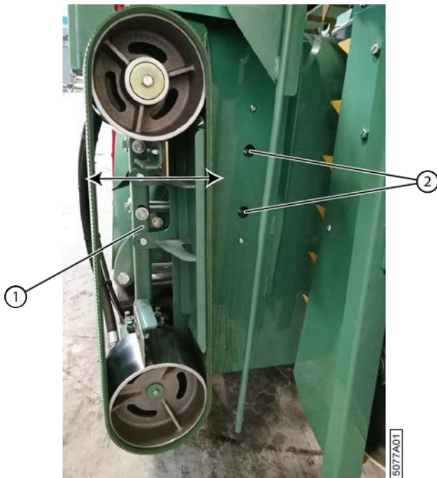
Fig. 97: Régler la courroie d'alignement coté pied
