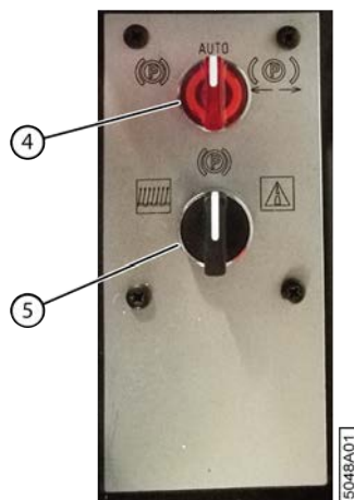
Fig. 67: Face inférieure de la console de commande
