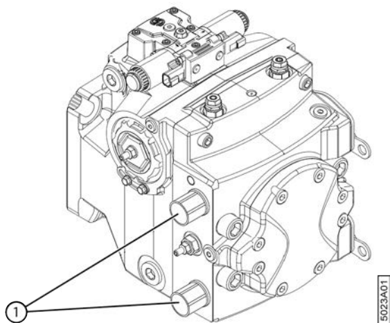
Fig. 118: Ouvrir le circuit hydraulique des roues
