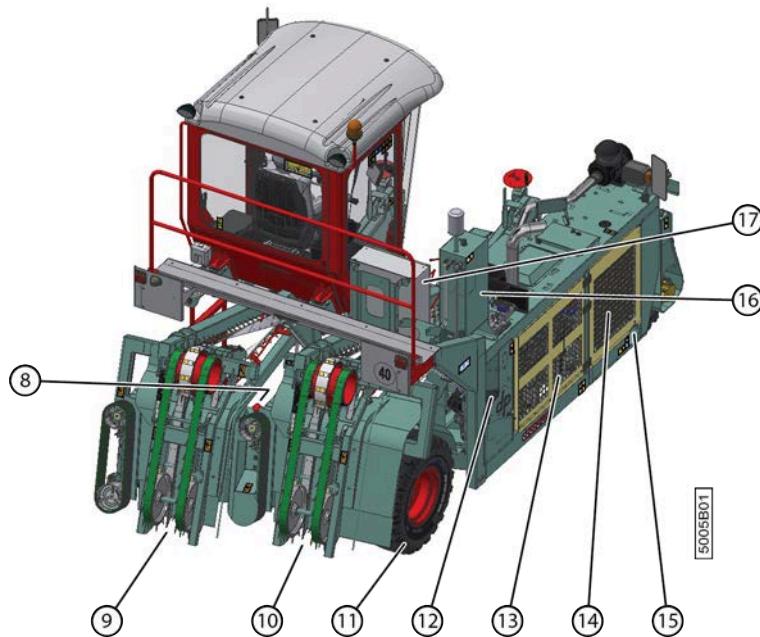
Fig. 9: Vue arrière
