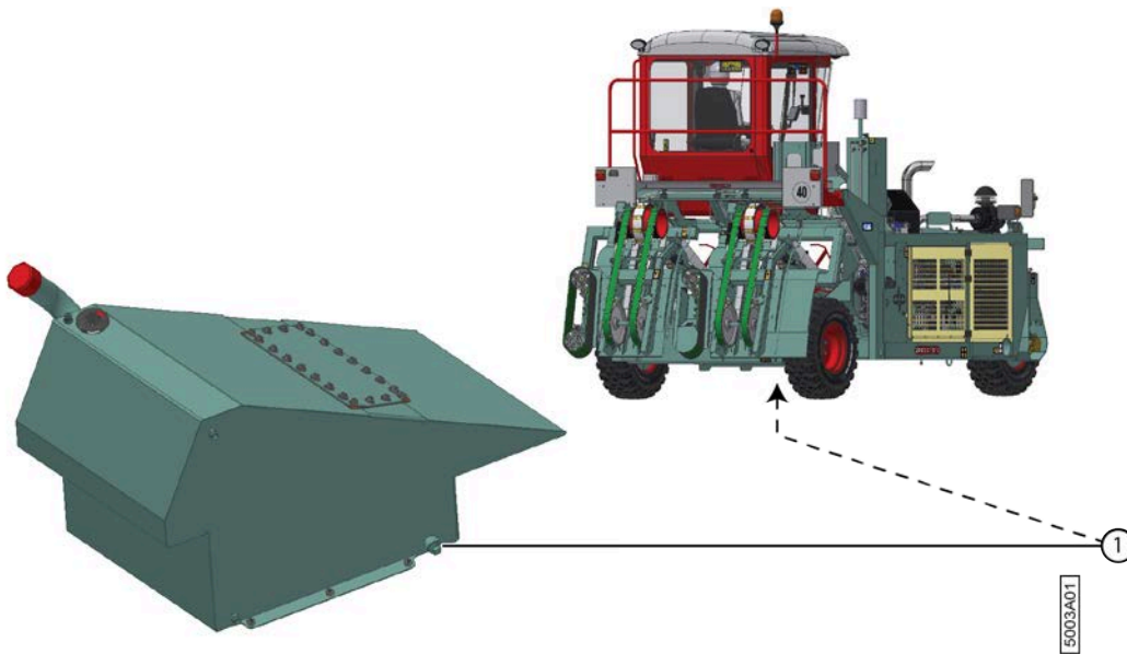
Fig. 134: Vidanger le réservoir à carburant
