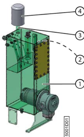
Fig. 108: Changer l'huile hydraulique
