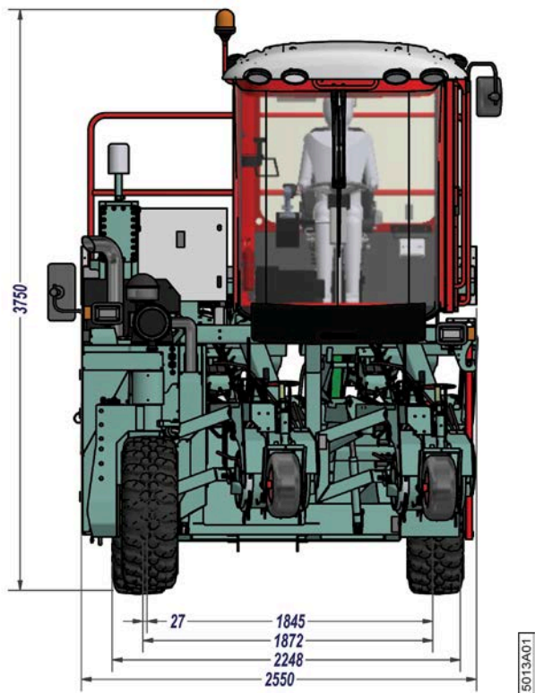
Fig. 5: Dimensions (largeur et hauteur)
