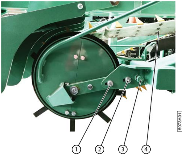
Fig. 89: Régler la tension des courroies
