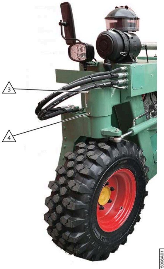
Fig. 112: Lubrifier la roue avant
