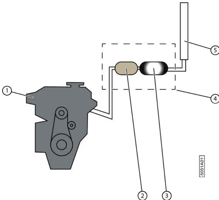
Fig. 129: Système de post-traitement des gaz d'échappement
