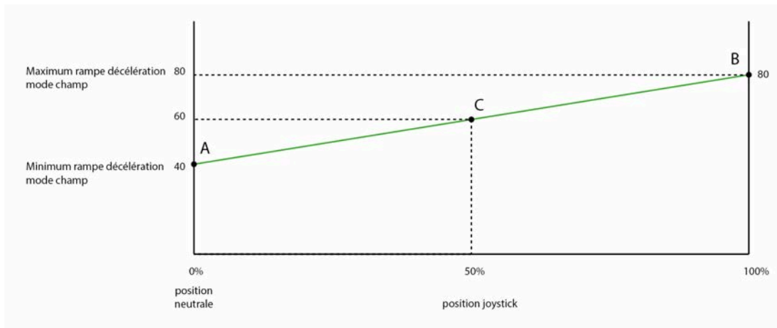
Fig. 79: Exemple de ralentissement en mode champs alors que la vitesse de réaction est réglée sur variable
