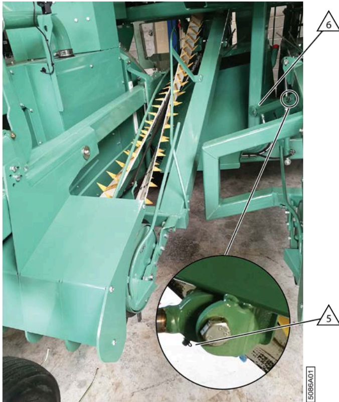
Fig. 113: Lubrifier le vérin du pick-up gauche
