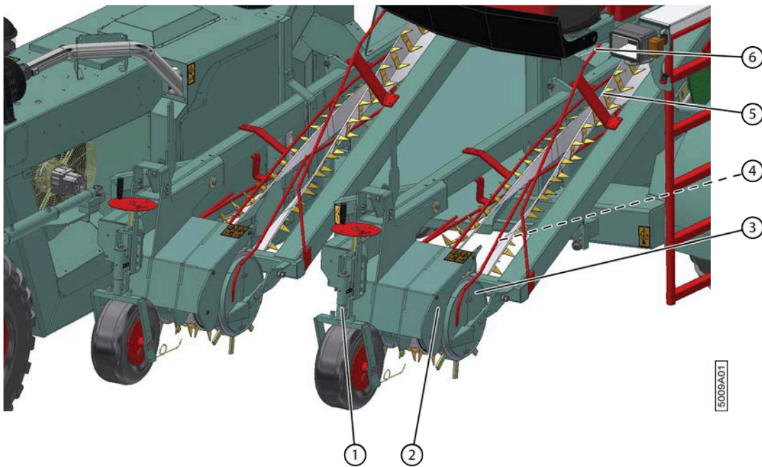
Fig. 33: Pick-up
