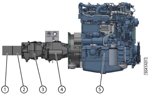
Fig. 35: Moteur + pompes hydrauliques
