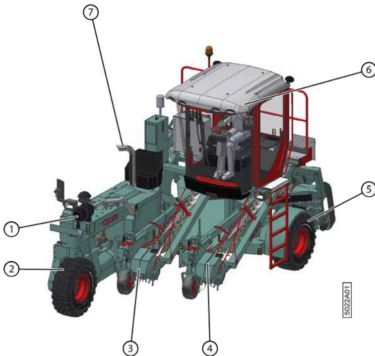
Fig. 8: Vue de face de la machine
