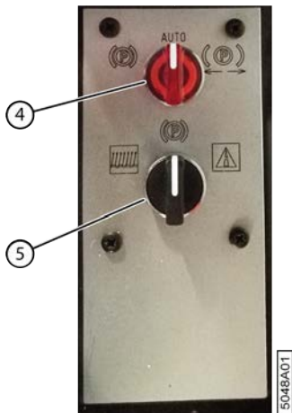
Fig. 65: Face inférieure de la console de commande
