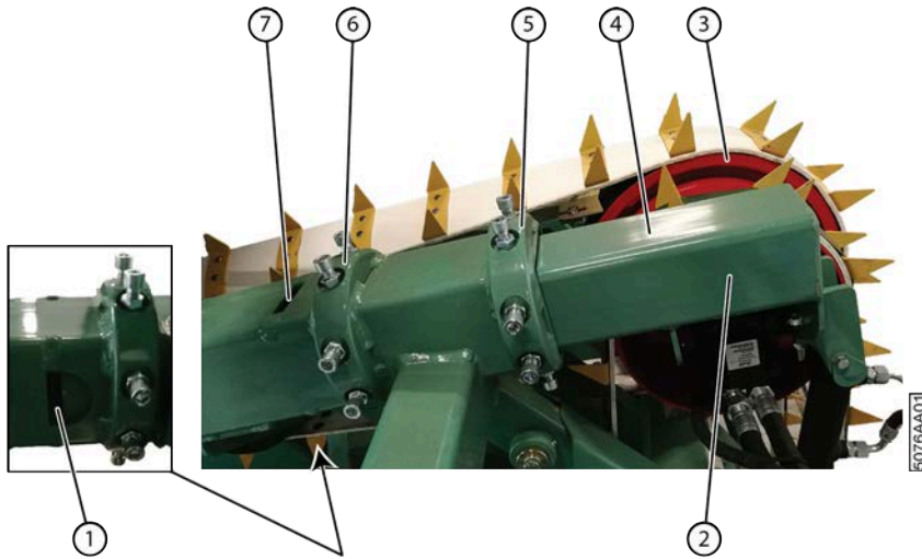
Fig. 94: Régler la roue motrice
