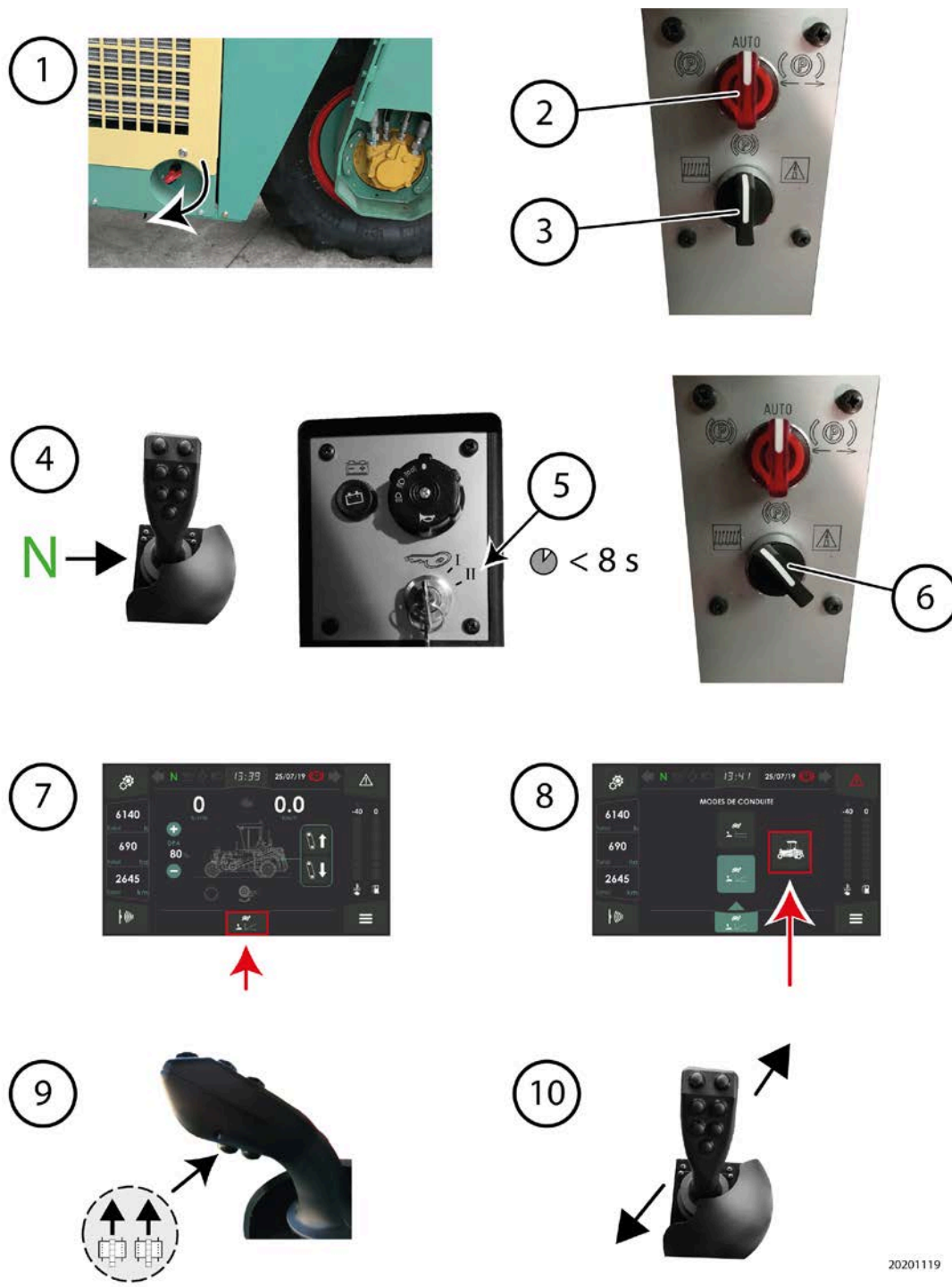
Fig. 45: Étapes de la descente
