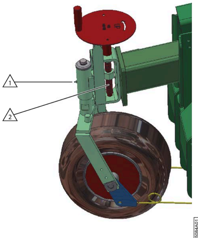
Fig. 111: Lubrifier la roue de jauge
