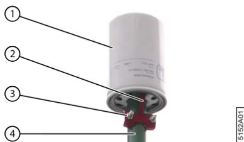
Fig. 109: Reniflard du réservoir hydraulique
