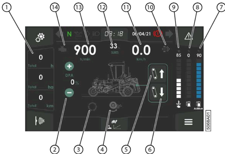
Fig. 66: Fenêtre mode champs
