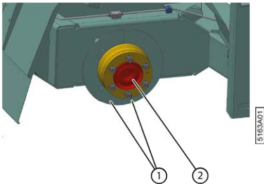
Fig. 114: Protections anti-salissure sur la roue droite
