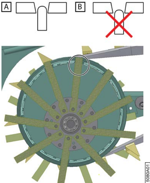
Fig. 103: Les dents du pick-up
