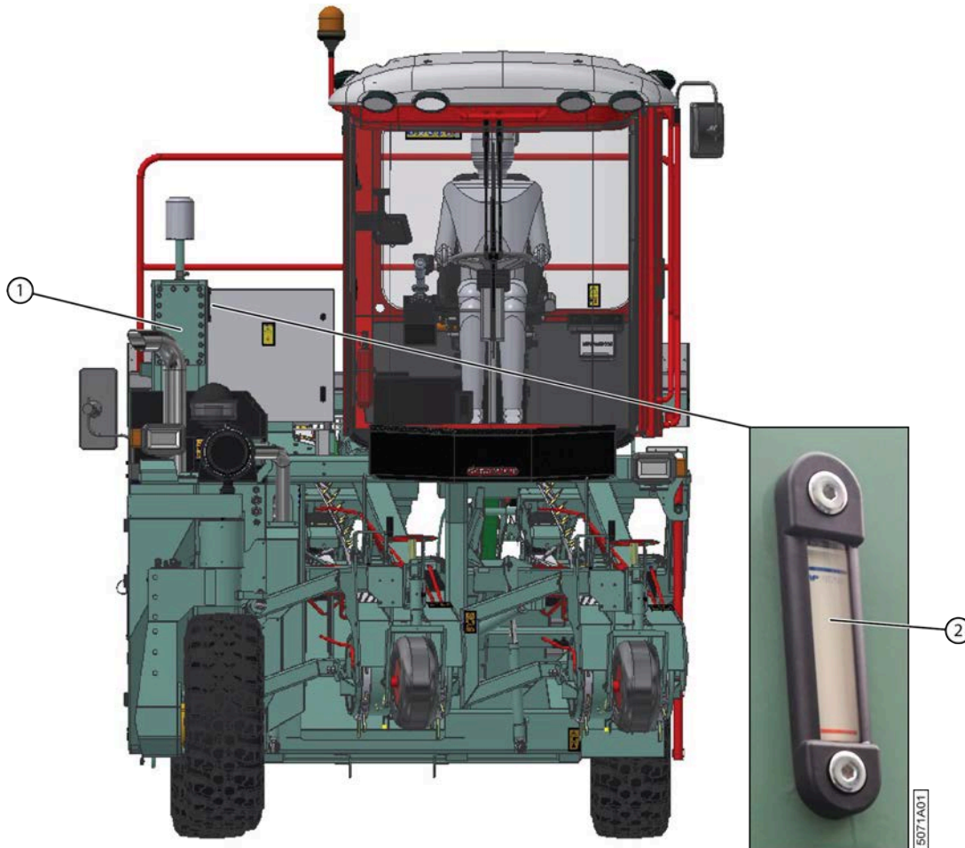
Fig. 107: Niveau huile hydraulique
