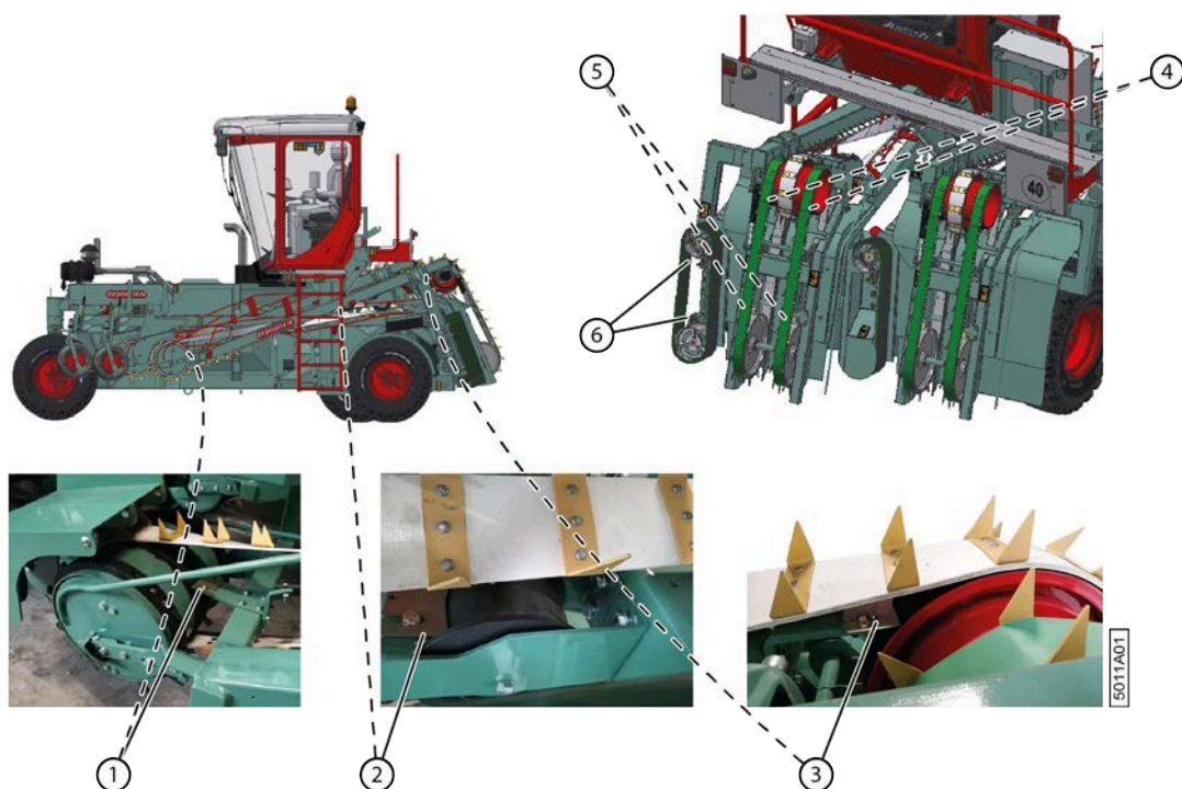
Fig. 91: Emplacement des racleurs
