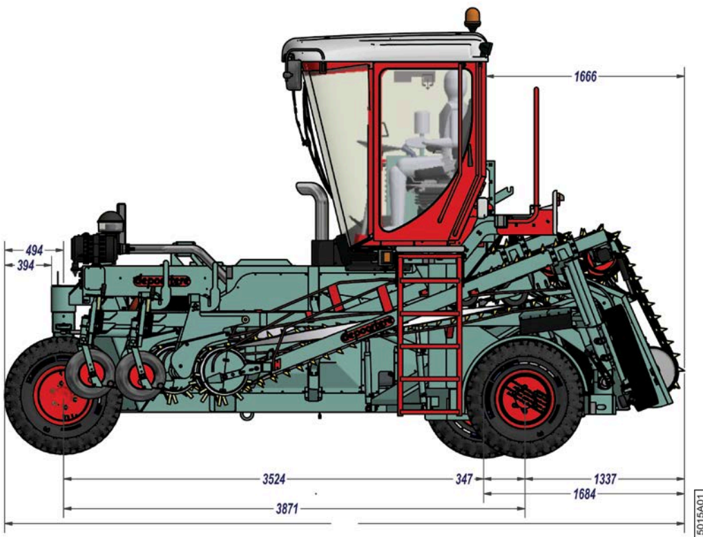
Fig. 6: Dimensions : longueur
