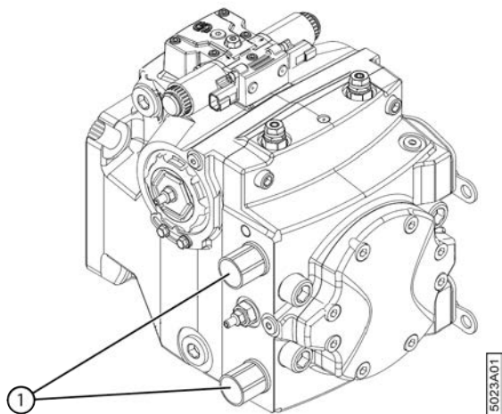
Fig. 116: Ouvrir le circuit hydraulique des roues
