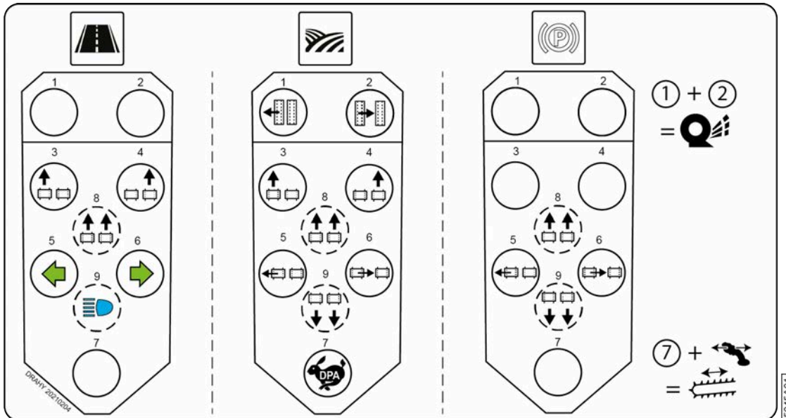
Fig. 48: Aperçu visuel des fonctions du joystick
