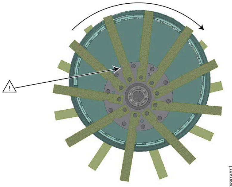
Fig. 125: Placement d'une nouvelle dent
