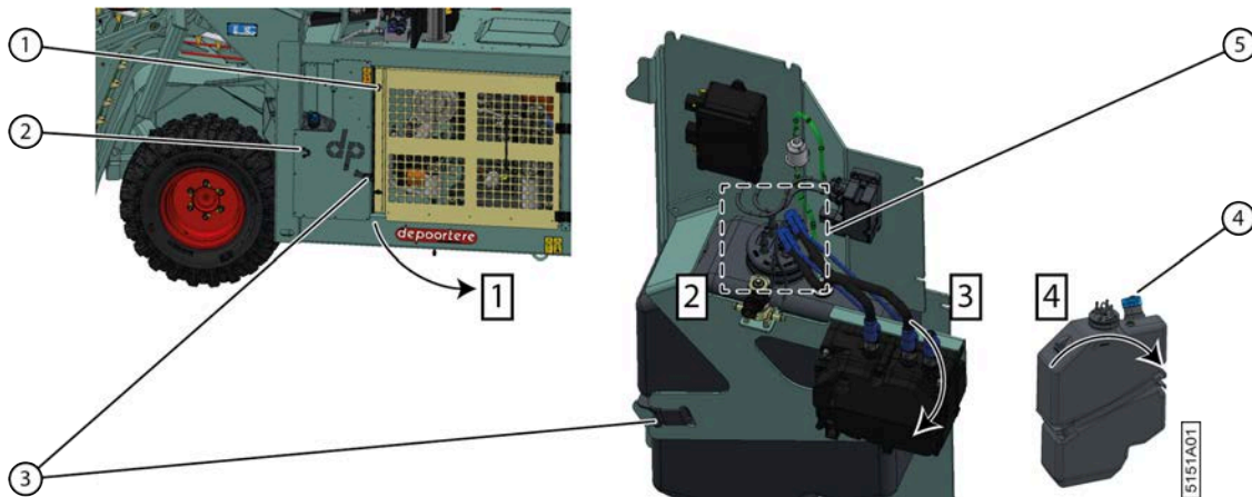
Fig. 46: Démontez et vidangez le réservoir d'AdBlue
