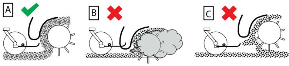
Fig. 85: Réglages possibles de la hauteur du pick-up
