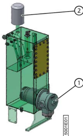
Fig. 141: Filtres sur le réservoir hydraulique
