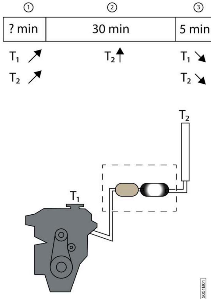
Fig. 130: Les 3 phases d'une régénération après arrêt
