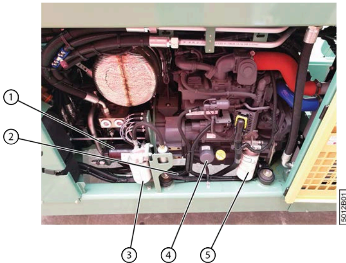
Fig. 138: Filtres dans le compartiment moteur
