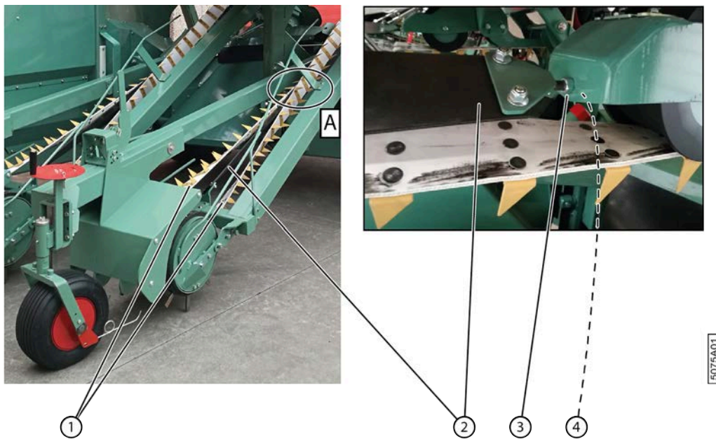
Fig. 93: Régler la tension de la courroie intermédiaire.
