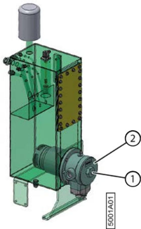
Fig. 100: Filtre d'aspiration réservoir hydraulique
