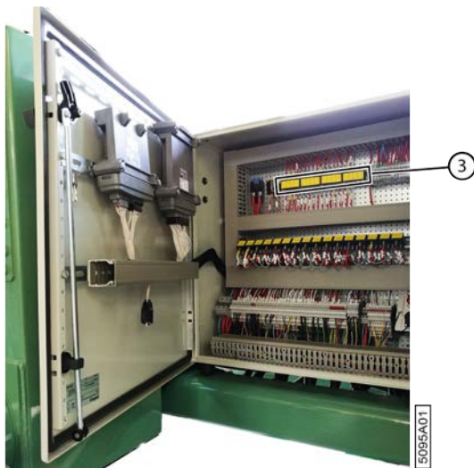
Fig. 128: Remplacer un fusible dans l'armoire électrique
