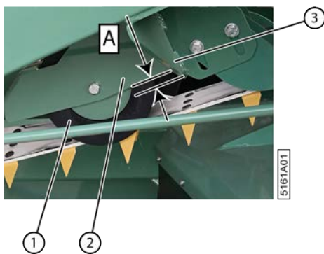
Fig. 95: Régler le galet de roulement d'une courroie de transport
