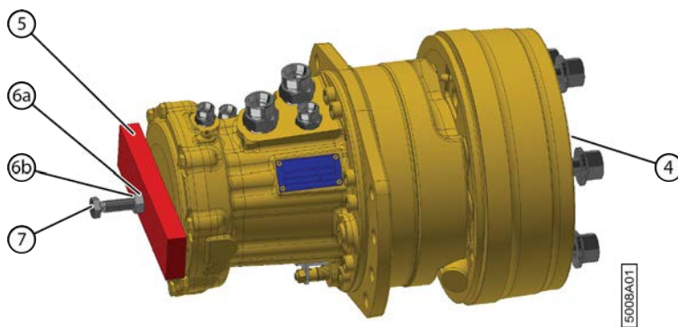
Fig. 119: Ouverture du frein
