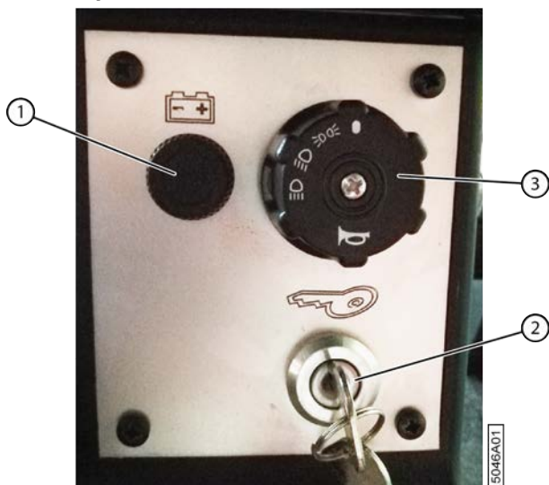
Fig. 49: Face supérieure de la console de commande
