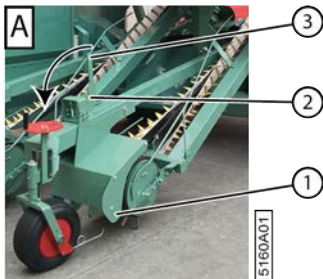
Fig. 77: Ouvrir le contre pick-up
