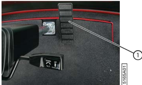
Fig. 51: Pédale de frein
