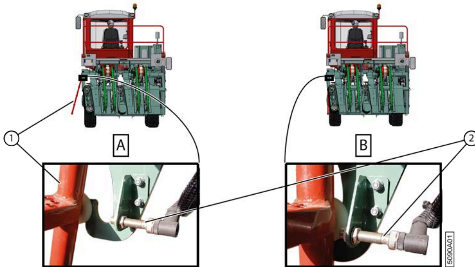
Fig. 12: L'échelle dépliée [A] et repliée [B].
