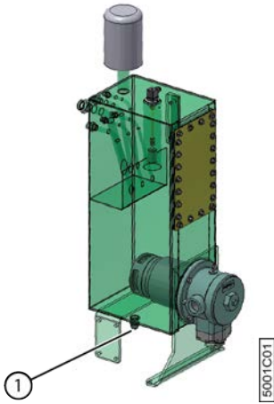
Fig. 133: Vider le réservoir d'huile hydraulique
