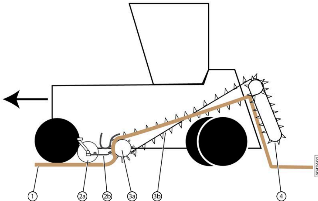
Fig. 38: Fonctionnement de la double retourneuse automotrice hydraulique
