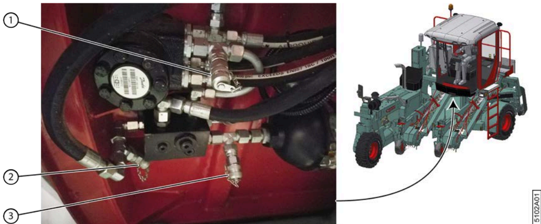
Fig. 131: Sous la cabine
