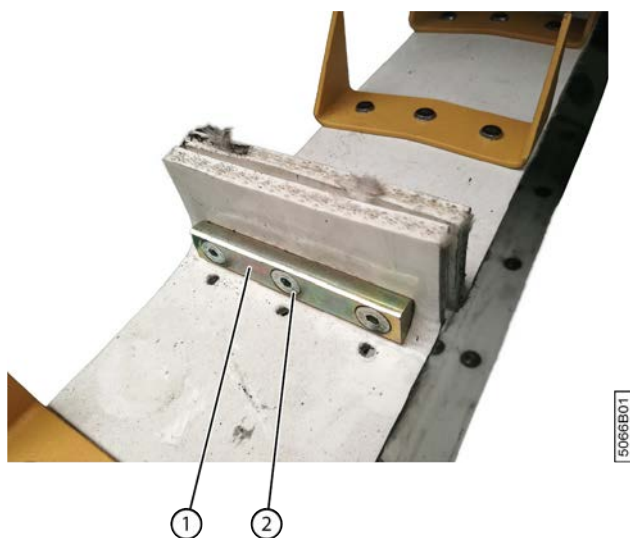
Fig. 123: Remplacer une courroie de transport
