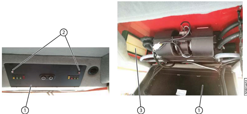
Fig. 105: Filtre à air dans le plafond de la cabine
