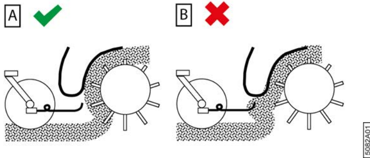
Fig. 87: Réglages possibles de la roue de jauge
