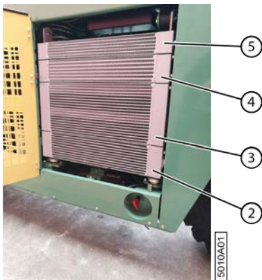
Fig. 36: Radiateurs
