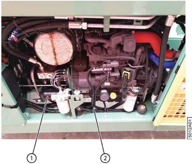
Fig. 99: Remplacer les filtres de pression de gavage
