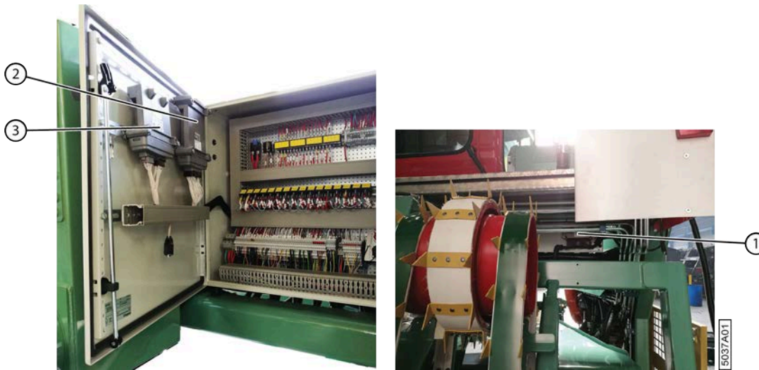
Fig. 30: Emplacement des contrôleurs
