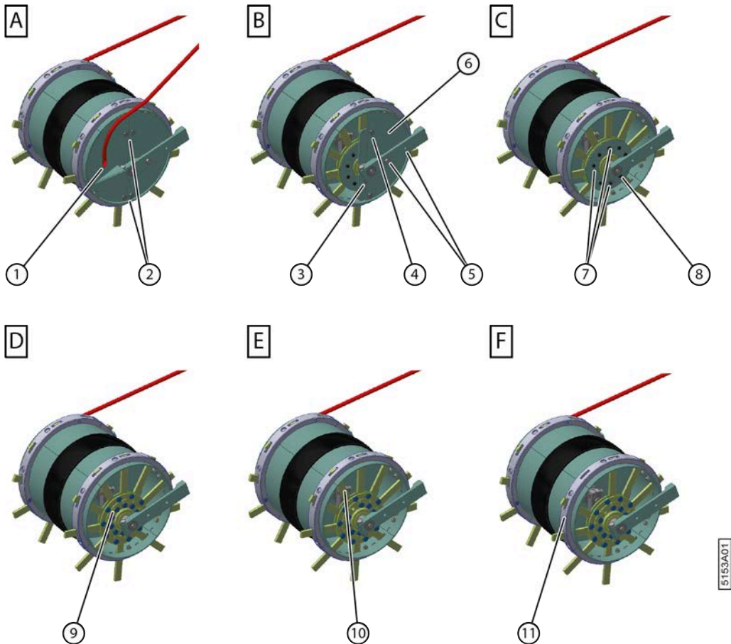
Fig. 124: Remplacer la dent du tambour de pick-up
