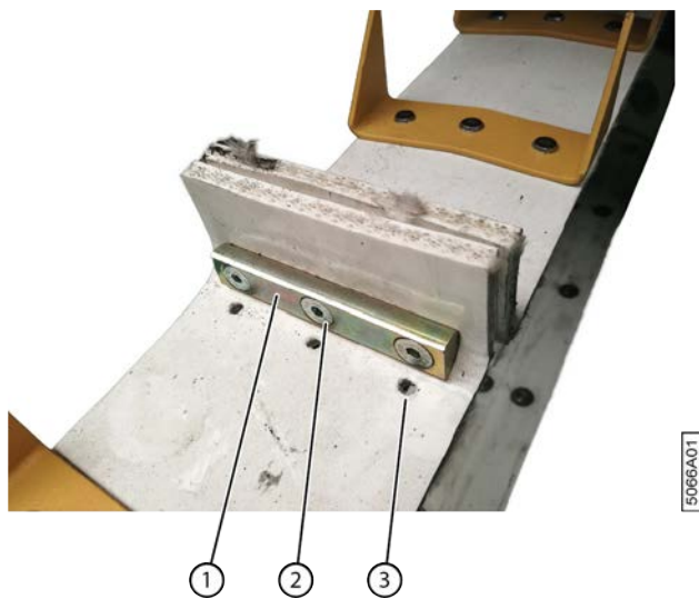
Fig. 90: Raccourcir les courroies de transport
