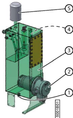
Fig. 28: Réservoir hydraulique
