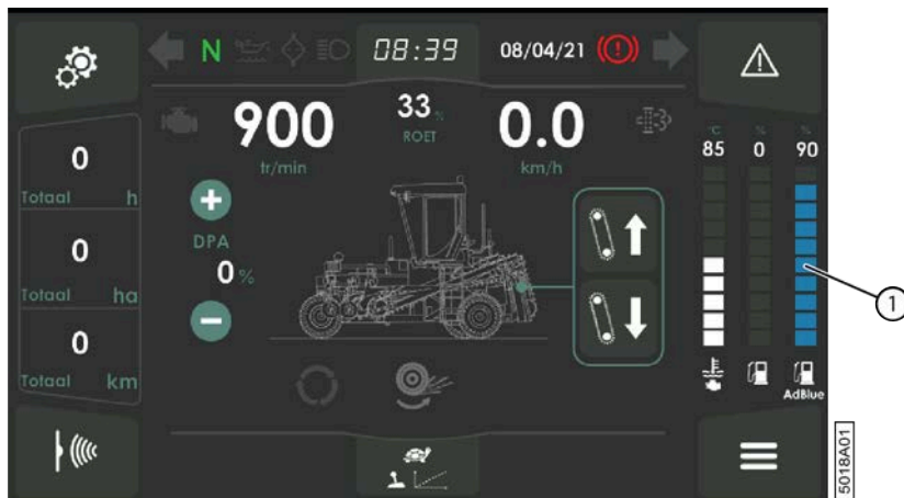
Fig. 57: Affichage du niveau AdBlue sur la fenêtre du mode champs
